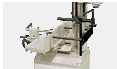
Set comprenant la butée et le dispositif de pression vers le bas pour un travail à 180° (No. d'art. 719 A-MDA)
